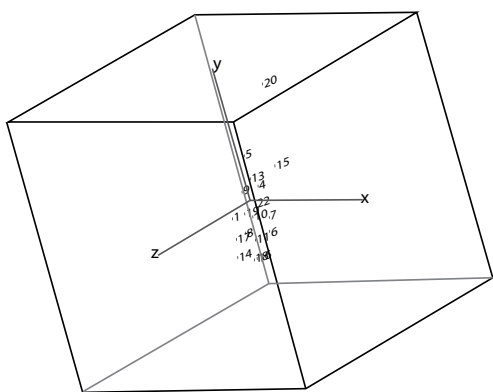
Figura 3. Ejemplo de rotación de la representación tridimensional que muestra la aproximación de los puntos a un plano referencial. Fuente: Villardon, 2002
