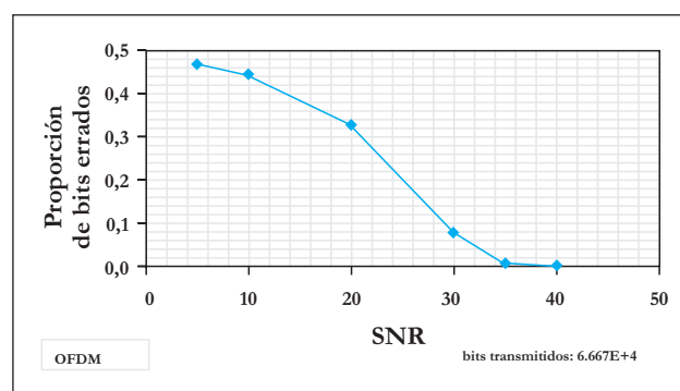
Figura 5. Relación señal a ruido vs proporción de bits errados tiempo de simulación OFDM .
