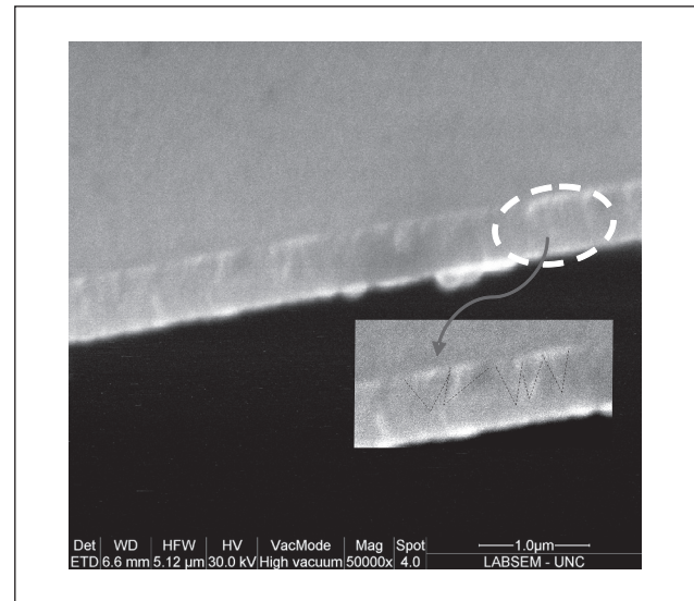
Figura 5. Micrografía de la sección transversal de la muestra de \mu\text{c-Si:H} intrínseca depositada sobre vidrio corning 7059. En el inset de la figura se muestra en forma ampliada la evidencia del crecimiento columnar marcada con línea a trazos.
