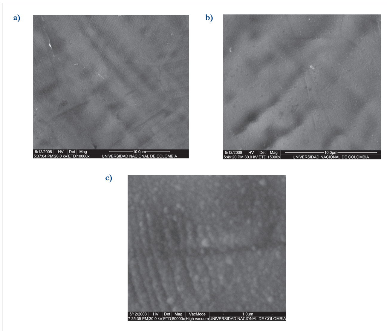
Figura 3. Micrografías SEM de muestras de Si depositadas sobre tres sustratos acero inoxidable. a) y b) corresponden a sustratos obtenidos comercialmente, y c) corresponde a acero inoxidable pulido previamente a la deposición.
