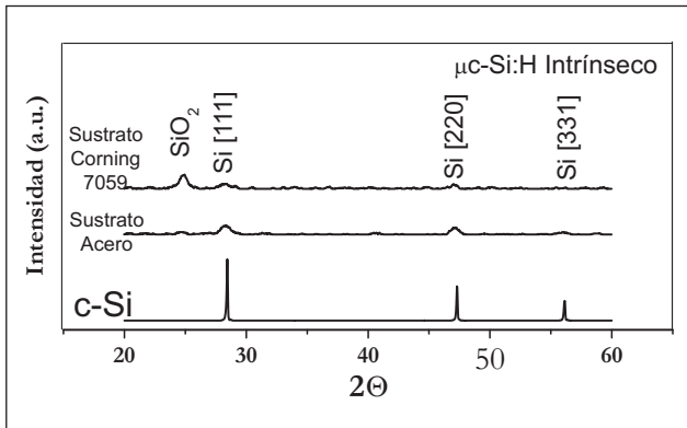
Figura 4. Espectro de XRD de muestras de silicio intrínseco depositada sobre sustratos de vidrio y acero inoxidable. Como referencia aparece el espectro típico del c-Si.
